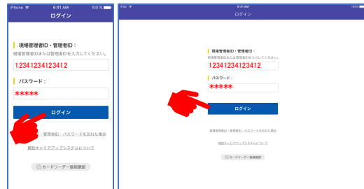
図 3-1 ログイン
